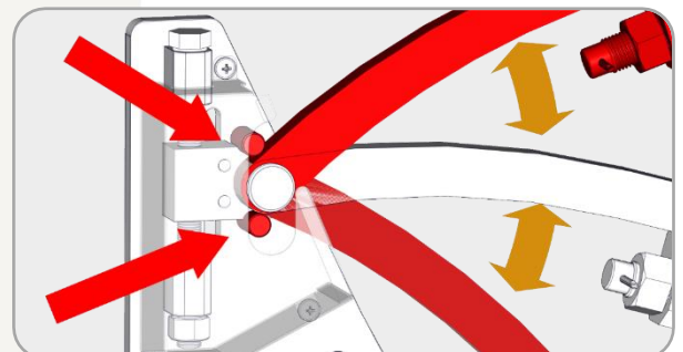
Figura 7 - Limite de Subida e Descida do Braço de Carregamento
