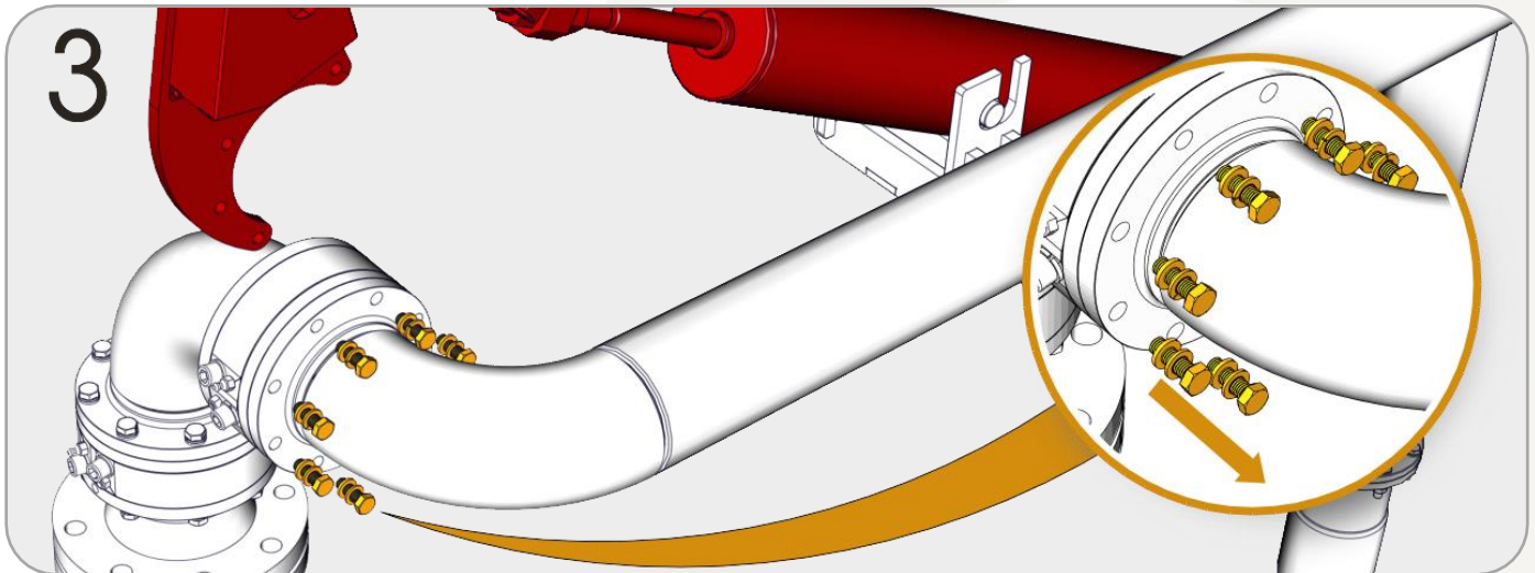
Figura 20 - Troca Vedações Junta Giratória 2- Passo 3
