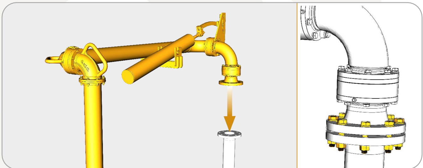
Figura 3 - Fixação do Braço de Carregamento no Flange de Entrada
