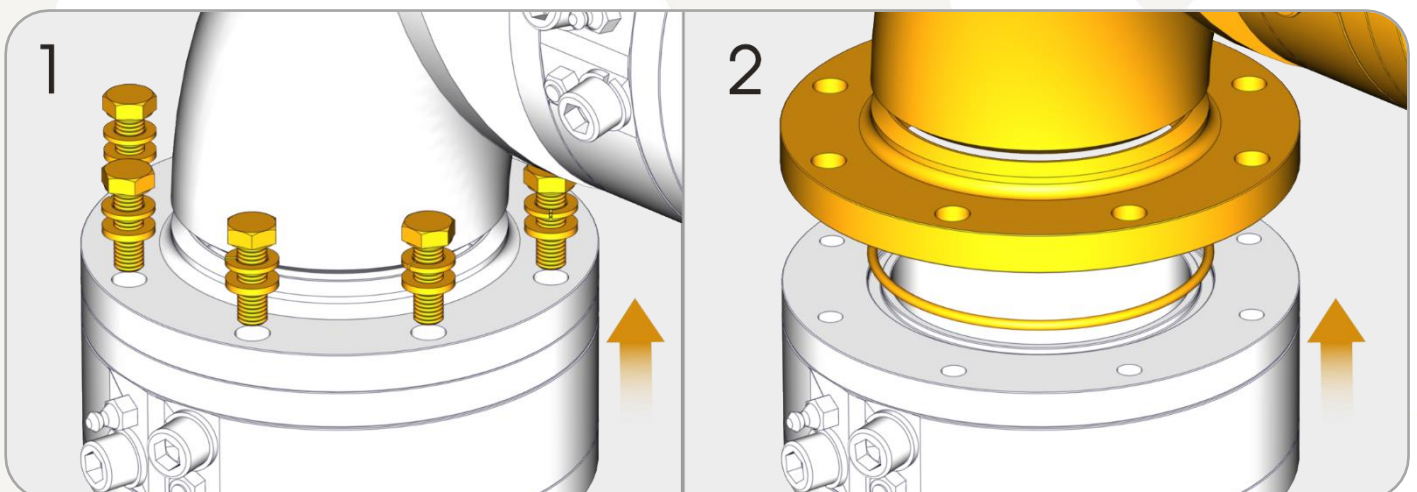
Figura 13 - Troca Vedações Junta Giratória 1- Passos 1 e 2
