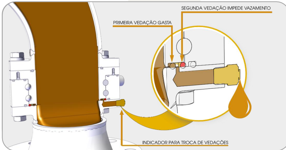
Figura 8 - Indicador para Troca de Vedação
