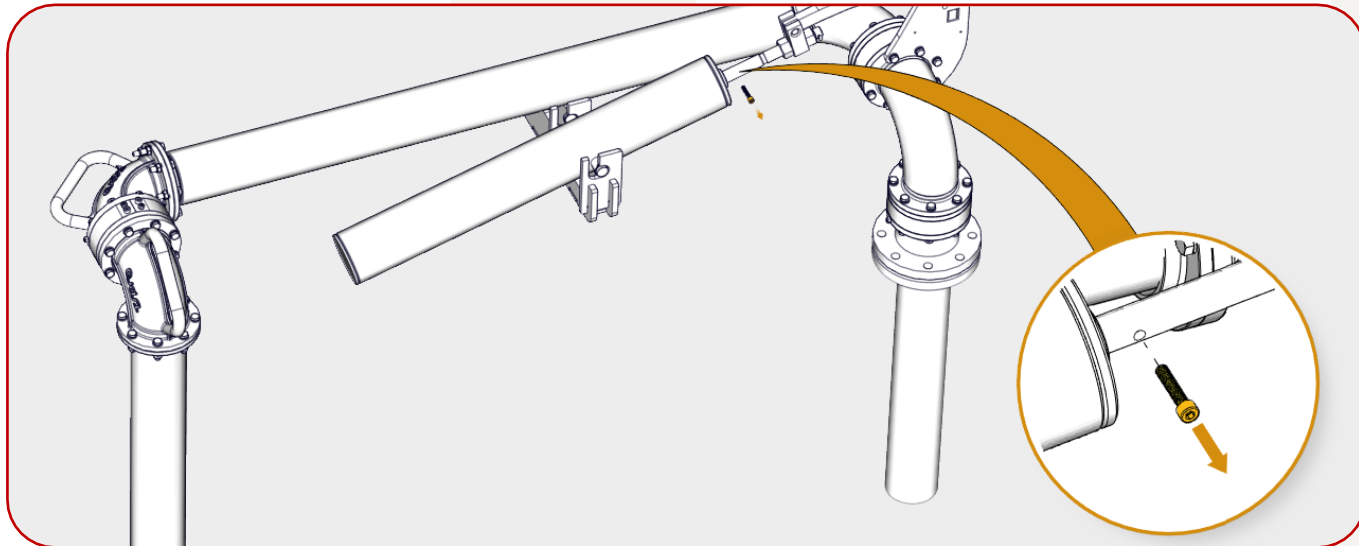
Figura 4 - Retirar o Parafuso de Trava do Conjunto de Mola
