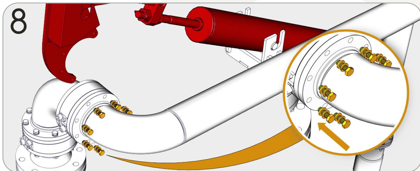
Figura 24 - Troca Vedações Junta Giratória 2- Passos 8
