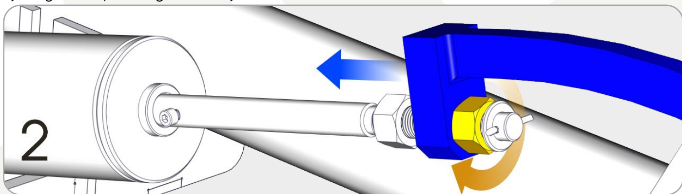
Figura 27 – Ajuste de Pré-Carga – Passo 2
