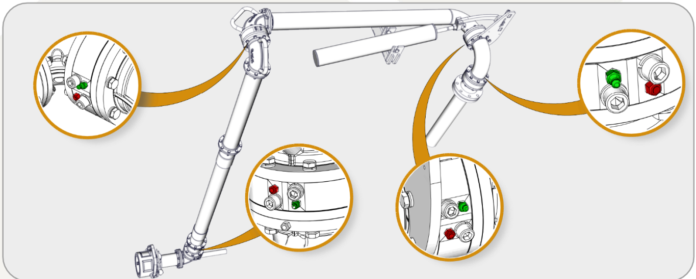
Figura 9 - Pontos de Engraxamento
