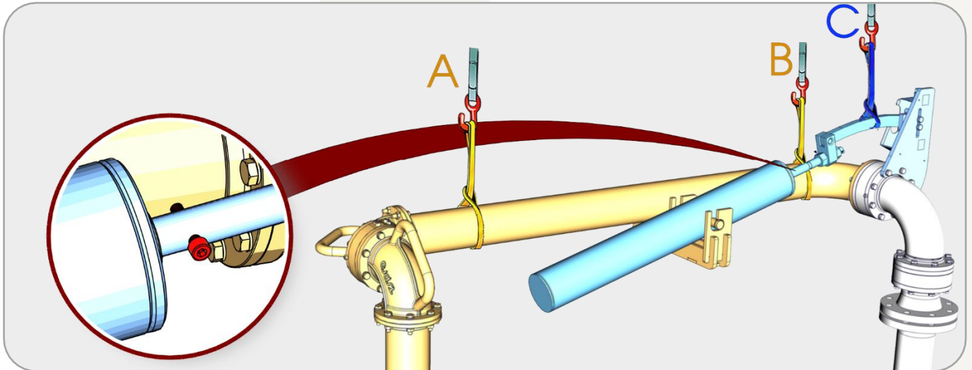
Figura 12 - Pontos de içamento
