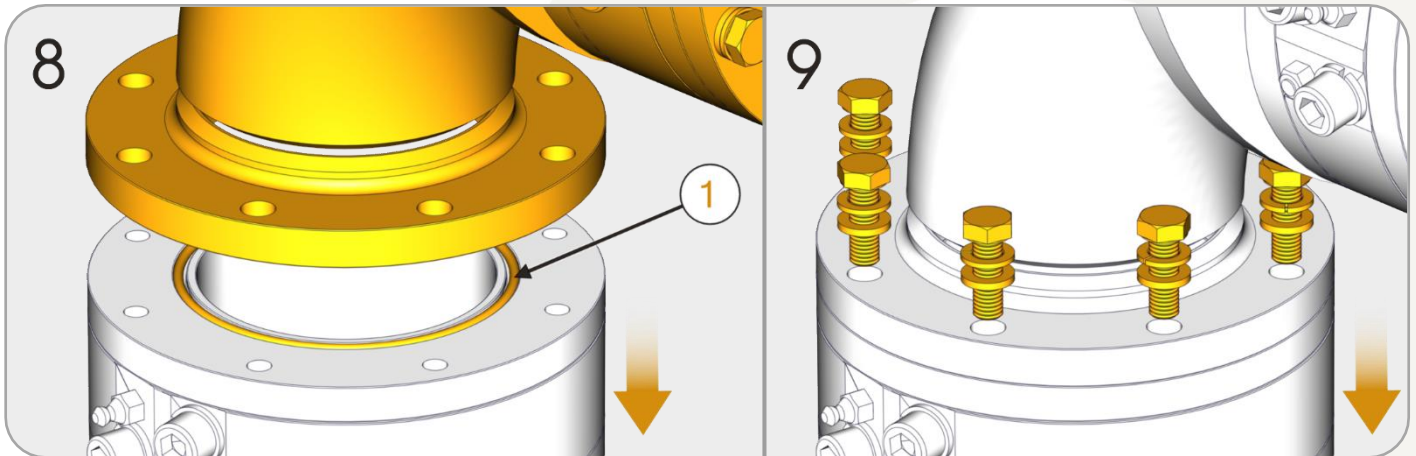
Figura 18 - Troca Vedações Junta Giratória 1- Passos 8 e 9
