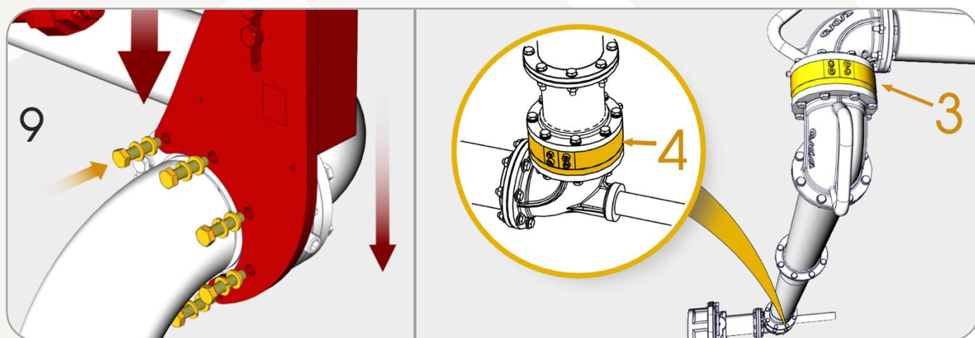
Figura 25 - Troca Vedações Junta Giratória 2,3 e 4- Passos 9 e 10
