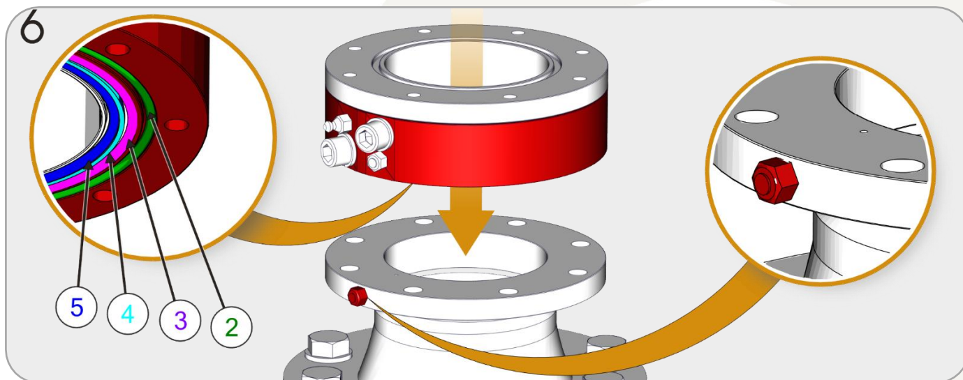
Figura 16 - Troca Vedações Junta Giratória 1- Passos 6
