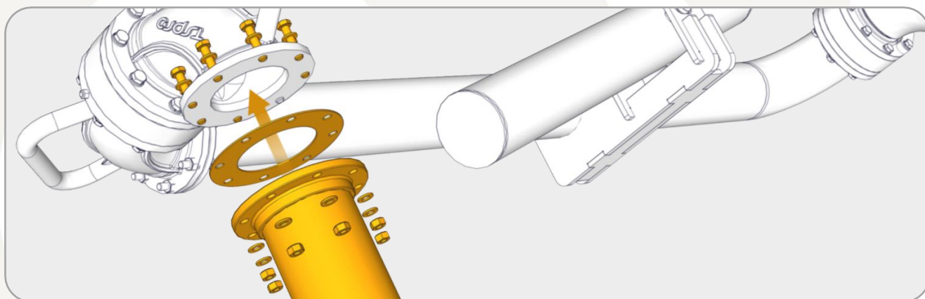
Figura 1 - Fixação Conjunto Mangueira Bottom
