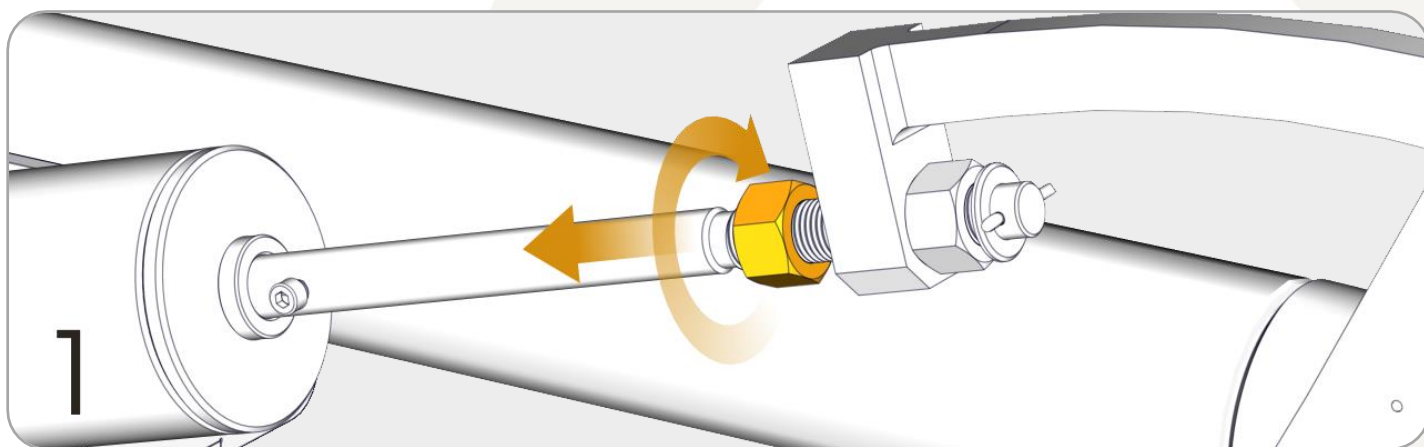
Figura 26 – Ajuste de Pré-Carga – Passo 1
