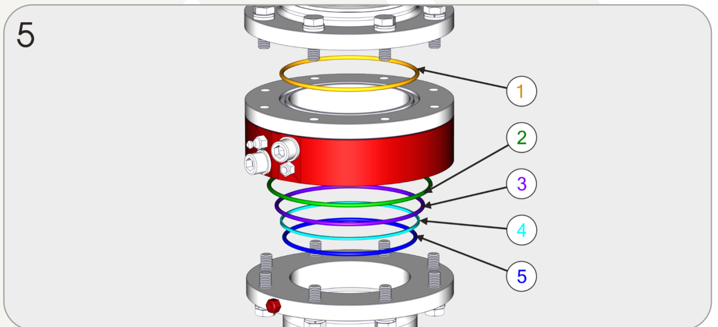
Figura 15 - Troca Vedações Junta Giratória 1- Passo 5
