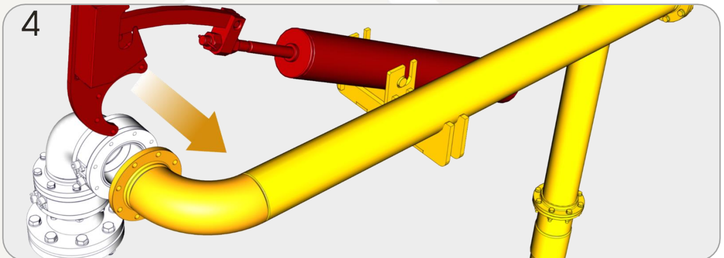
Figura 21 - Troca Vedações Junta Giratória 2- Passos 4
