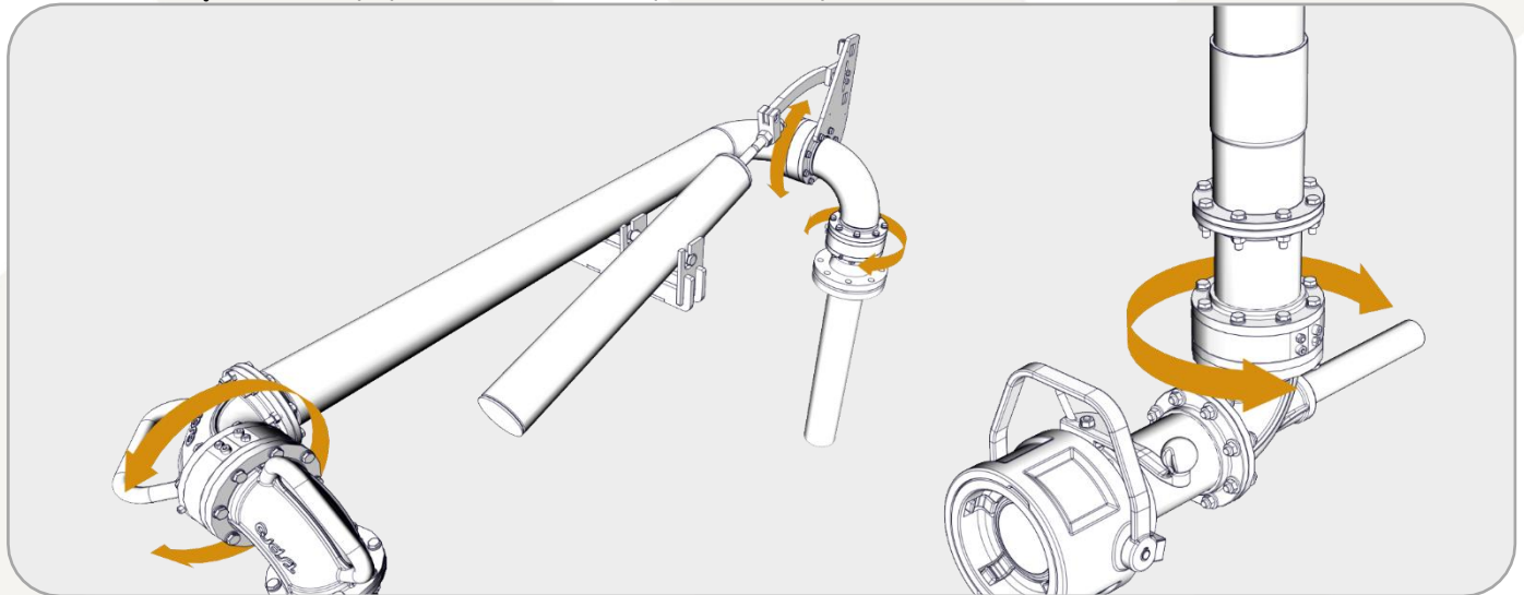
Figura 6 - Graus de Liberdade do Braço de Carregamento
