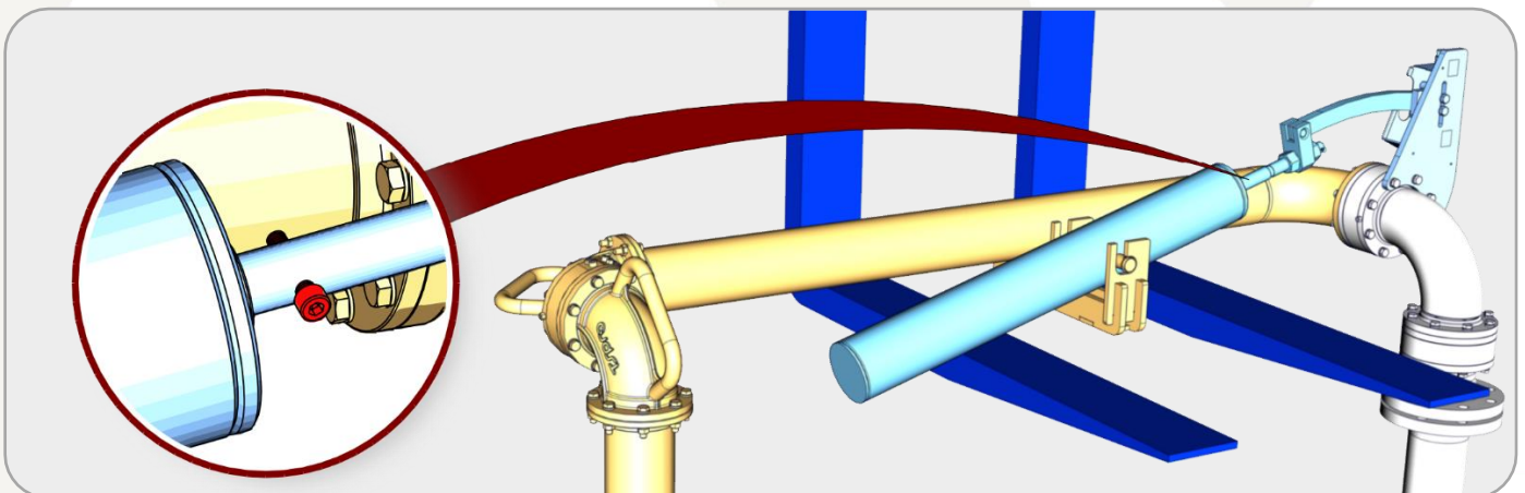
Figura 11 - Suspensão do Braço por Empilhadeira
