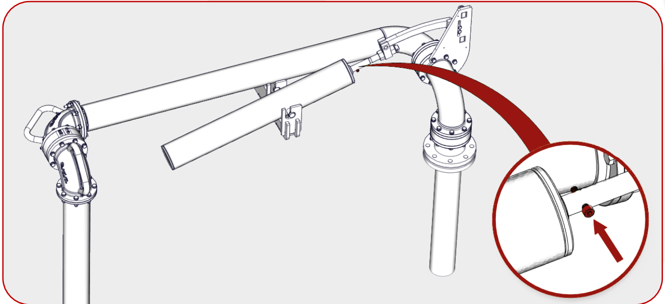
Figura 2 - Trava de movimentação do Conjunto de Mola
