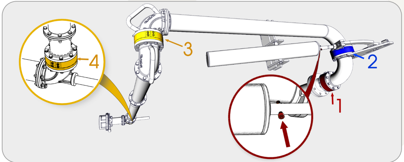
Figura 10 - Identificação das Juntas Giratórias e TRAVA DE SEGURANÇA
