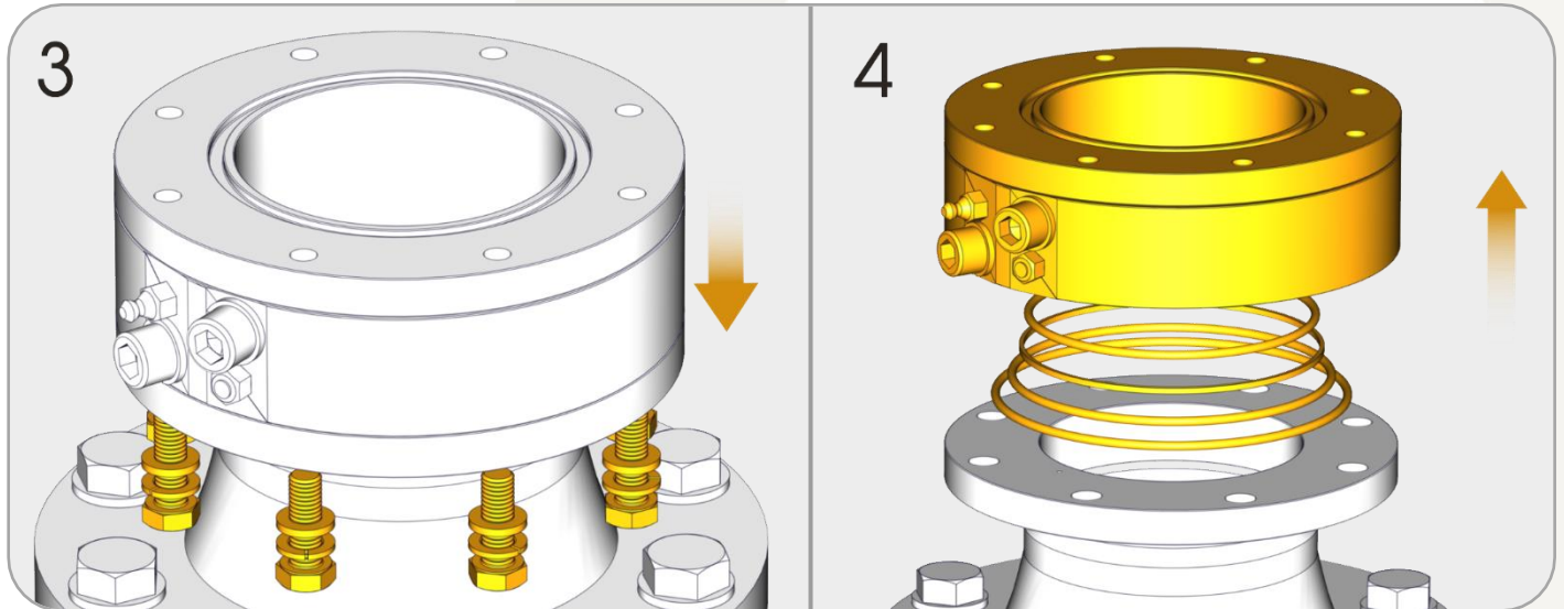
Figura 14 - Troca Vedações Junta Giratória 1- Passos 3 e 4
