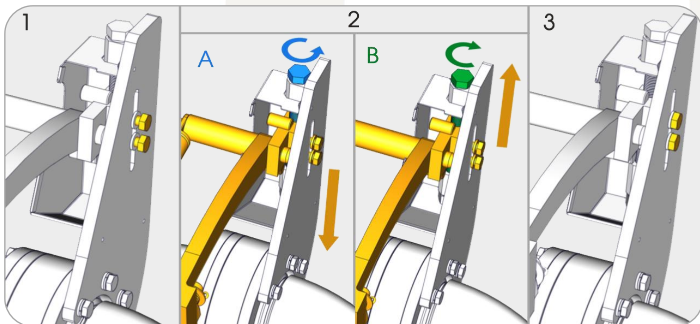
Figura 5 - Ajuste de Força da Mola
