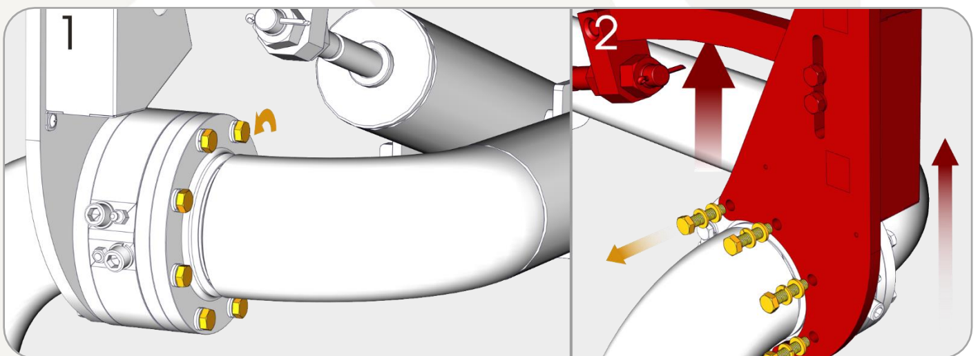
Figura 19 - Troca Vedações Junta Giratória 2- Passos 1 e 2
